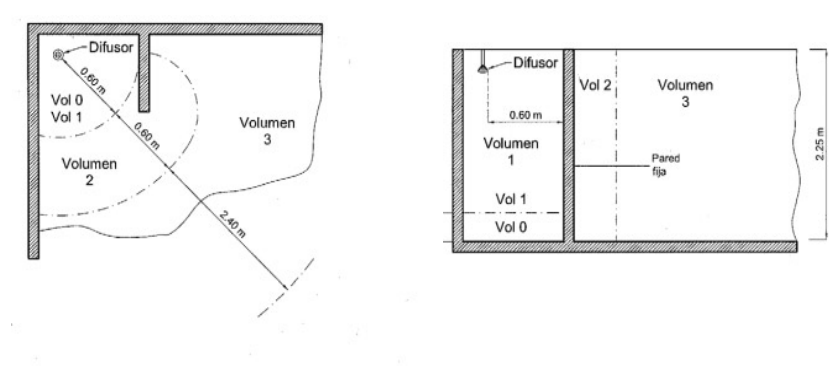
Figura 7 – CABINA DE DUCHA PREFABRICADA
