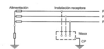
Figura 5. Esquema de distribución tipo IT
