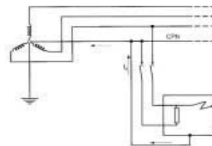
Figura 2. Esquema TN-C.
