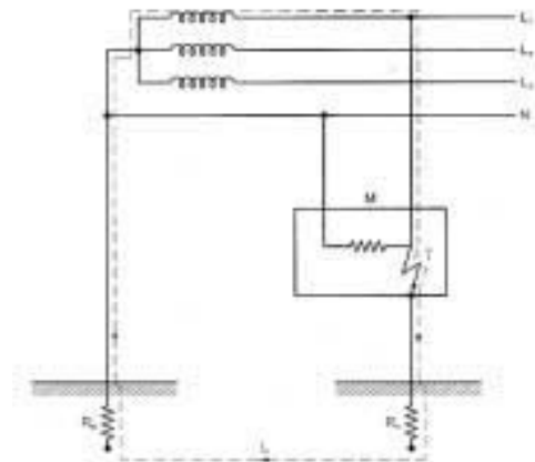
Figura 4 Esquema TT
