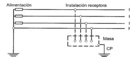
Figura 4. Esquema de distribución tipo TT
