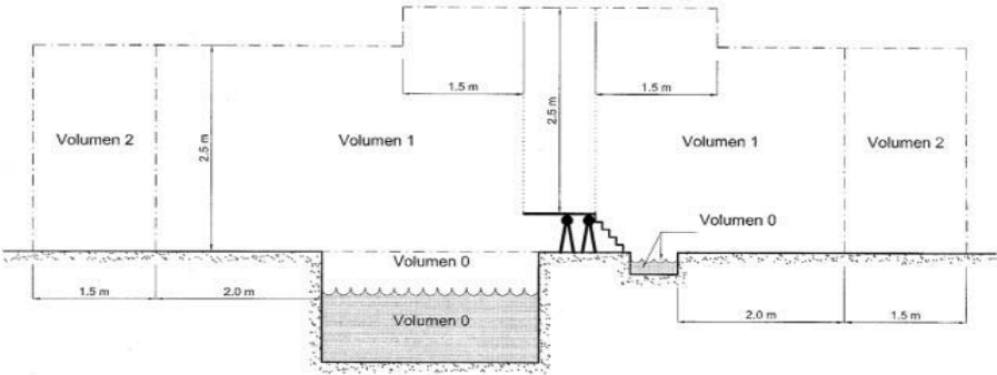
Figura 1. Dimensiones de los volúmenes para depósitos de piscinas y pediluvios
